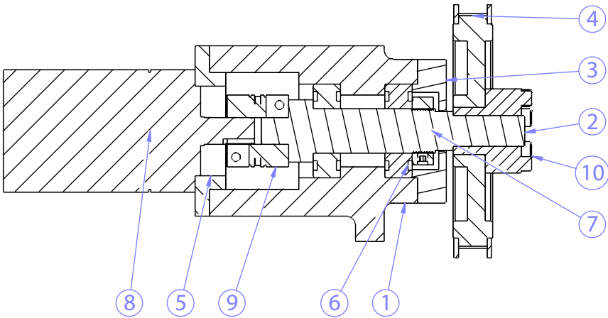
剖面圖 A-A
