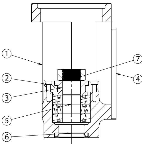
剖面圖 A-A
