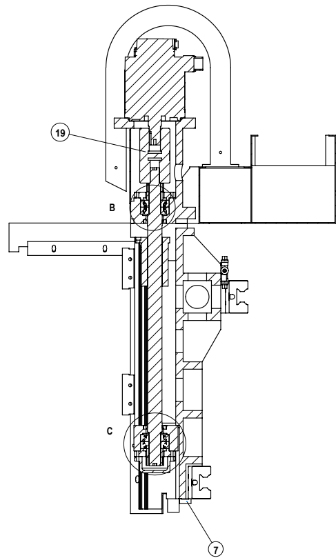
剖面圖 A-A
